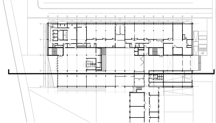
PLANTA BAJA
