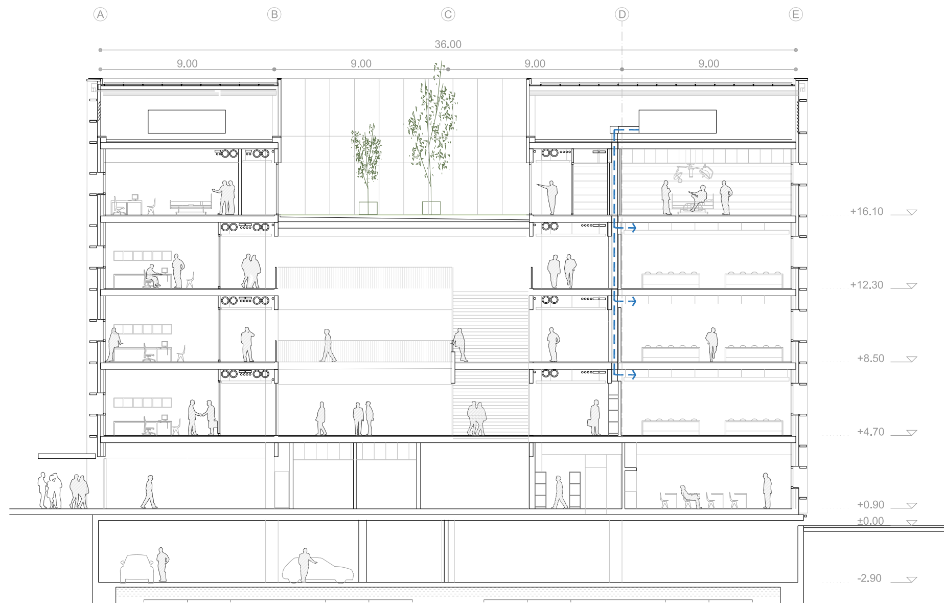
SECCION TRANSVERSAL 2
