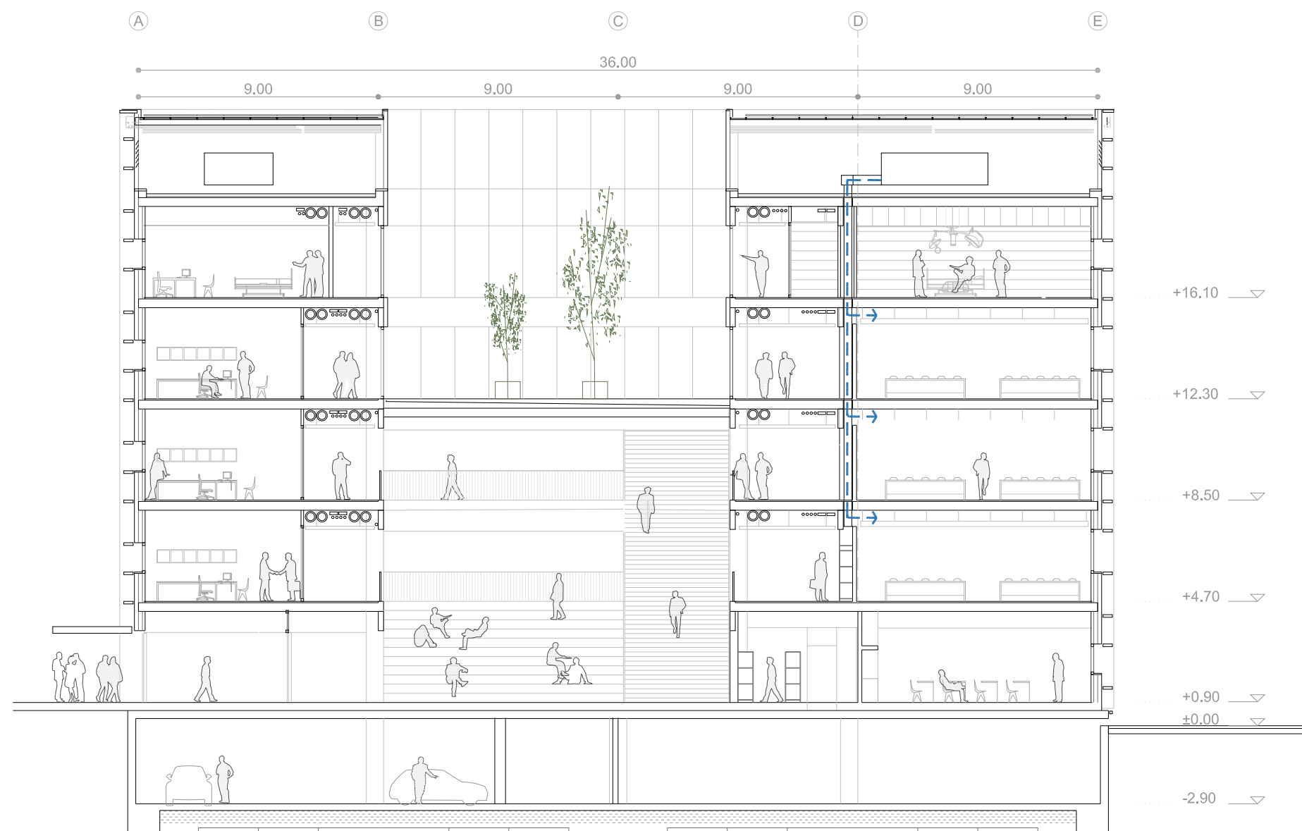
SECCION TRANSVERSAL 1
